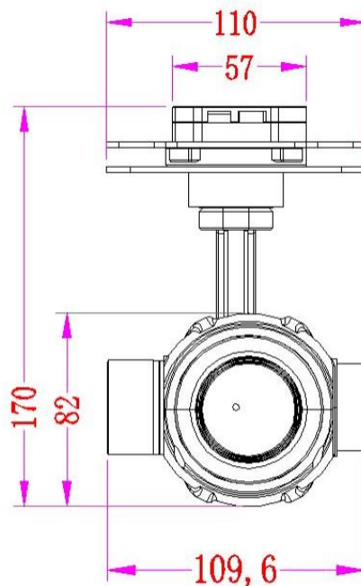
图 1-1-1 云台结构
