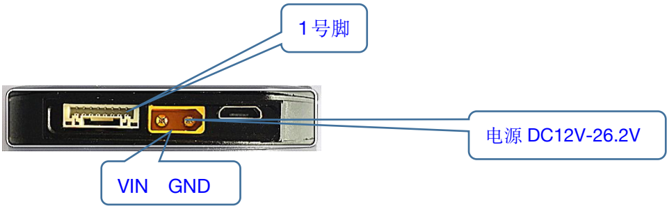
连接应用图
