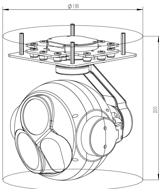
图 1-1-1 三光一体云台结构
